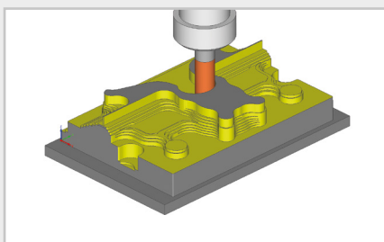
Simulace obrábění
